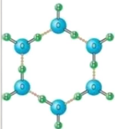
ЛЕД
