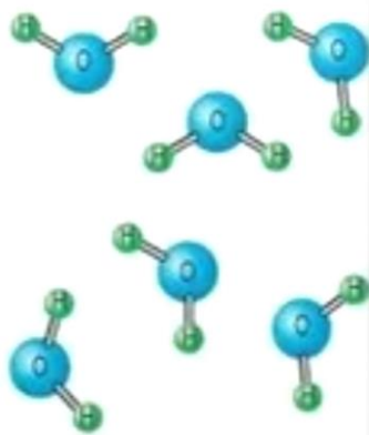
ПАР
