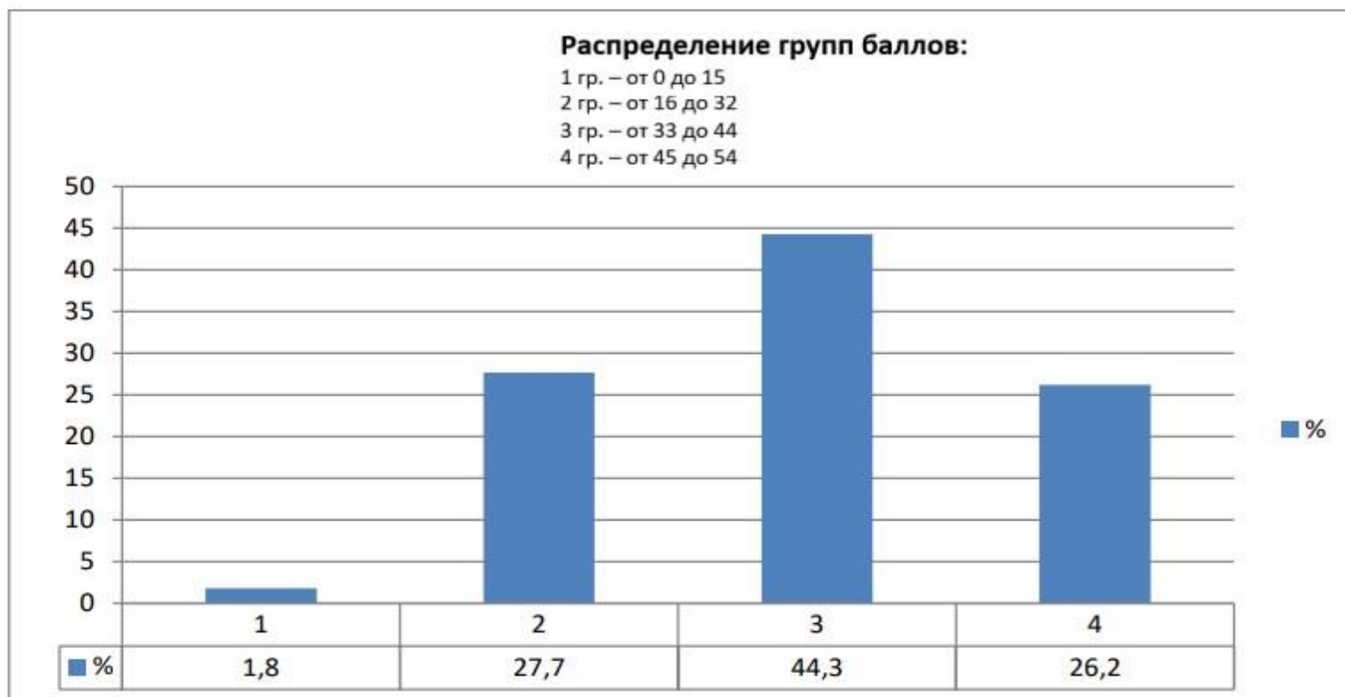
Рис. 3. Распределение участников ЕГЭ с различным уровнем подготовки по группам баллов
